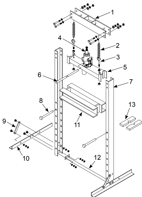
Figure 8 : Illustration des pièces de rechange du modèle 60120
