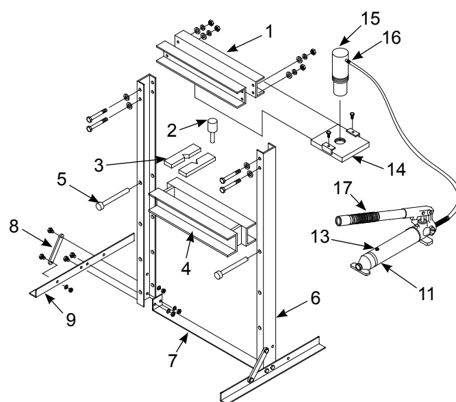
Figure 11 - Illustration des pièces du modèle 65123
