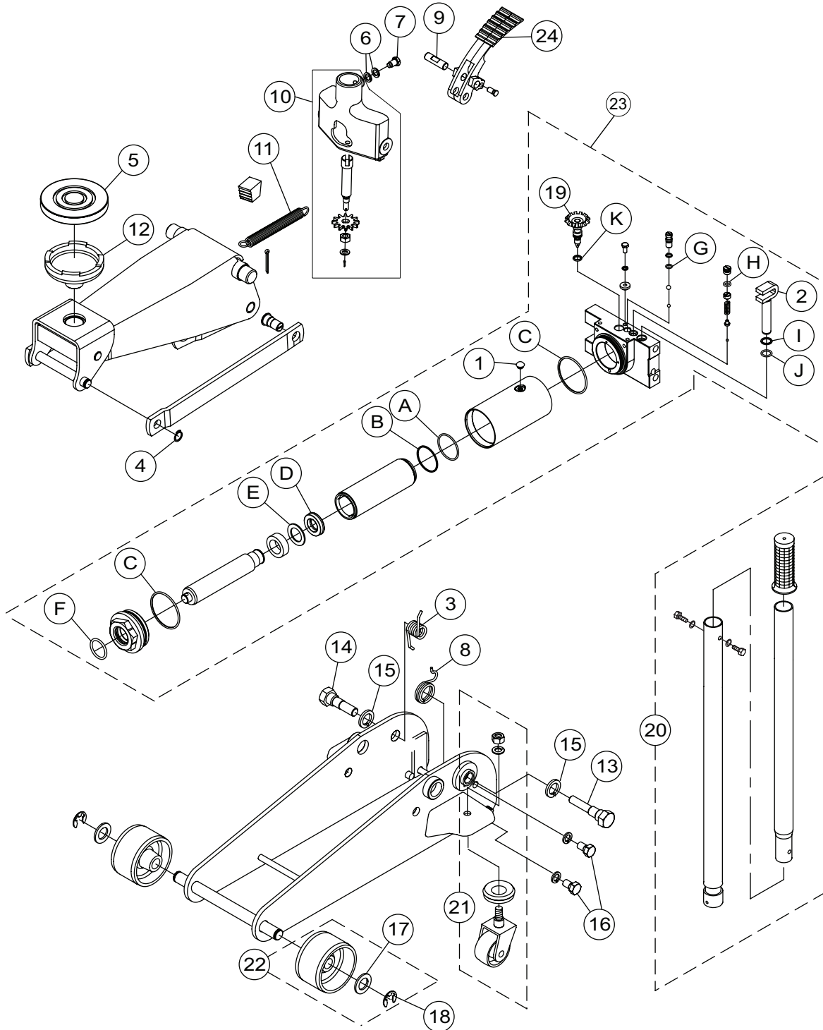
Figura 2: Ilustración de piezas de repuesto para el modelo BH6034B
