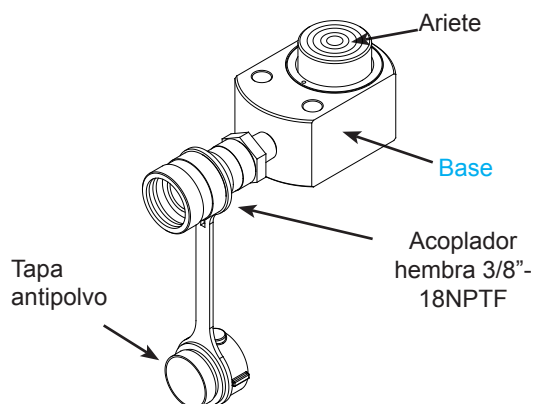
Figura 1: Componentes habituales del cilindro
