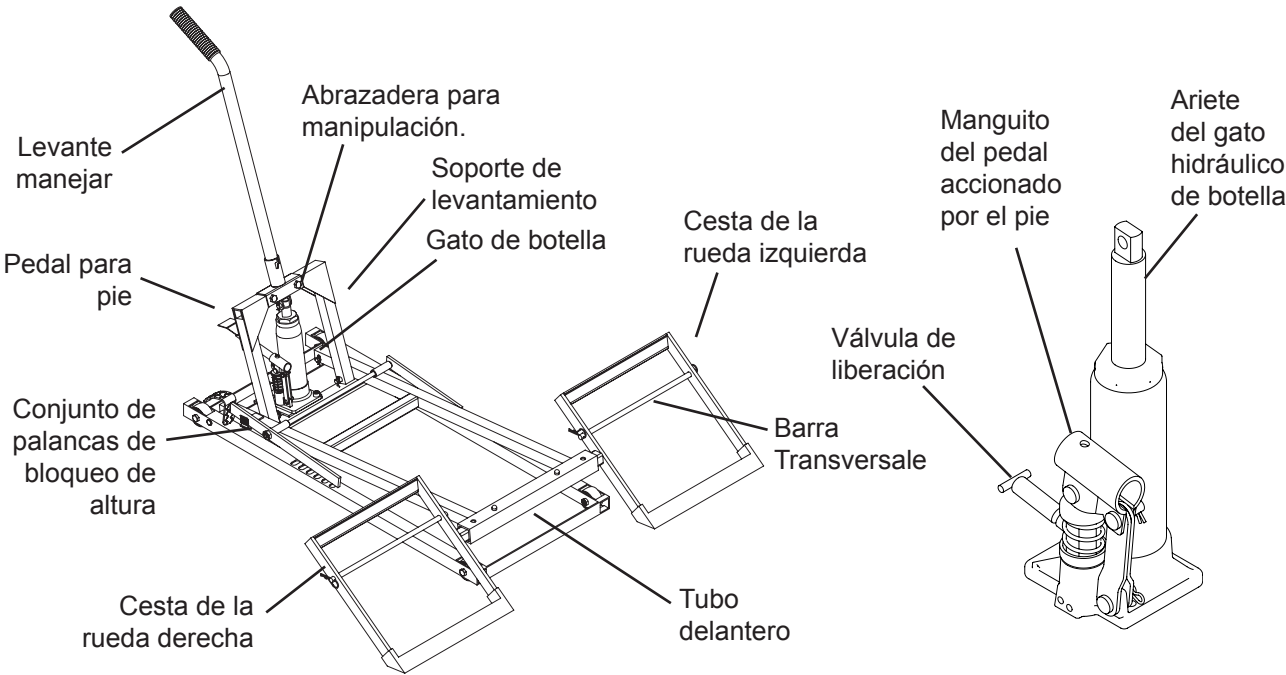
Figura 1: Nomenclatura de la elevadora.
